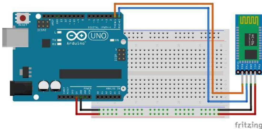
Figura 12.2. Esquema de conexión del Arduino a módulo bluetooth HC-06 de 4 pines.
