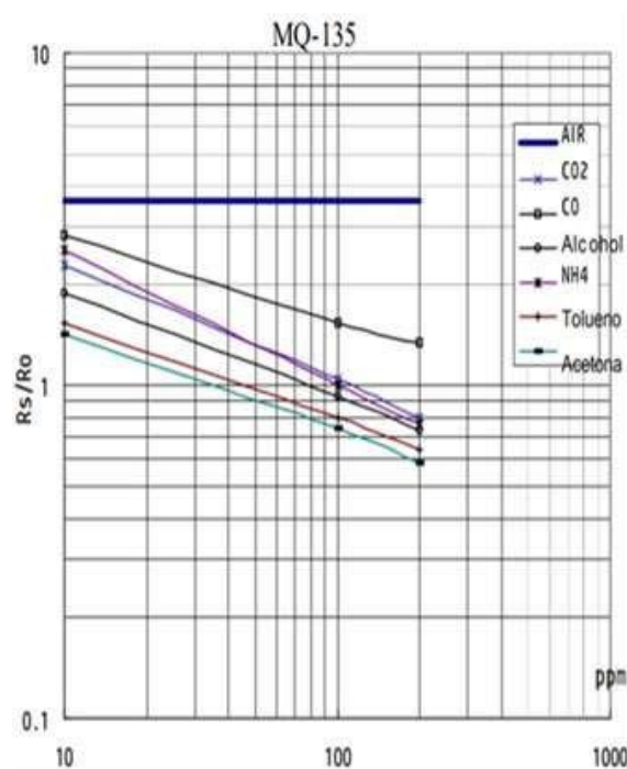
Figura 4. Curva característica del sensor MQ-135 según hoja de datos del fabricante.
