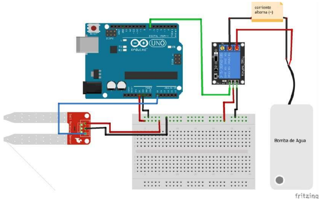
Figura 1. Esquema del circuito de riego automatizado.
