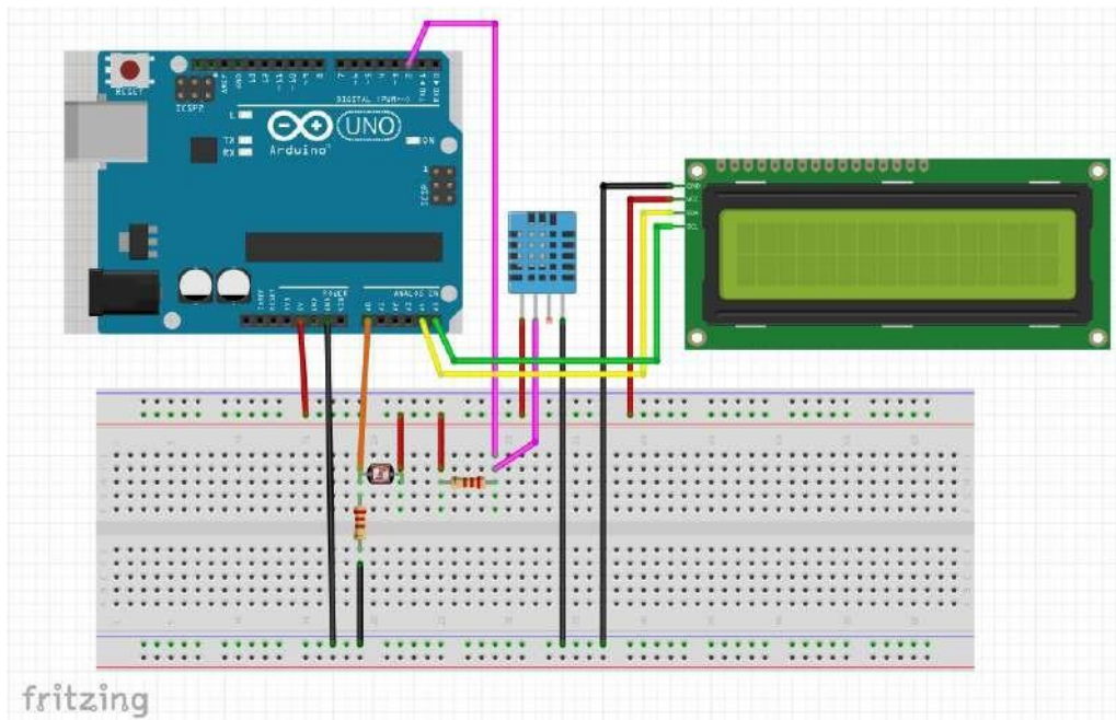
Figura 1. Esquema de circuito de microestación de monitoreo ambiental.
