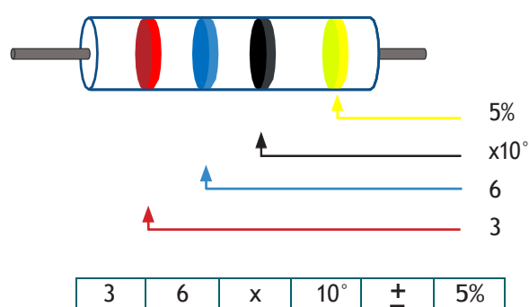
Figura 2.2. Esquema código de colores para resistencia de 36Ω.
