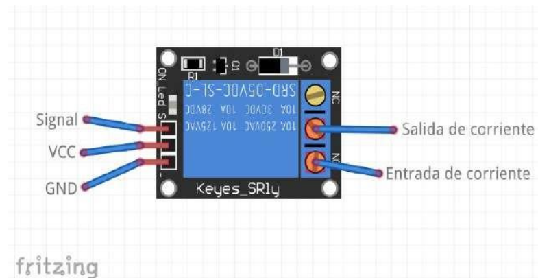
Figura 4. Conexiones principales del relé.
