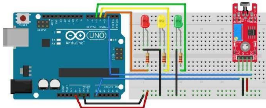
Figura 1. Circuito sonómetro con semáforo.
