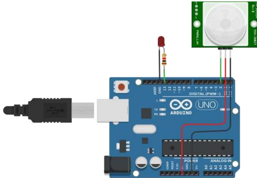
Figura 13.2. Circuito sensor PIR para activar un led
