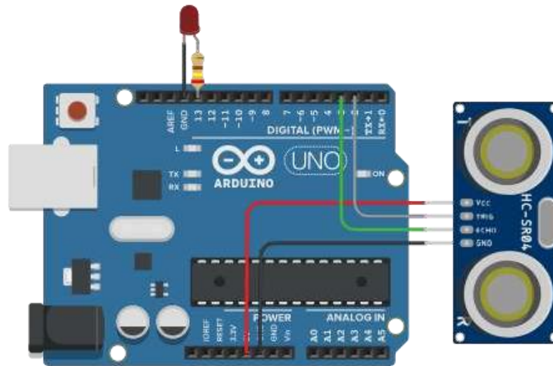
Figura 8.4. Montaje sugerido para trabajar el código HC-SR04 para medir distancia y controlar led.
