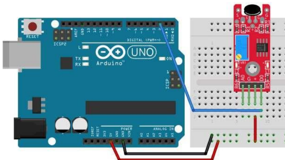
Figura 7.2. Circuito sensor ky-037 usando solo salida digital.
