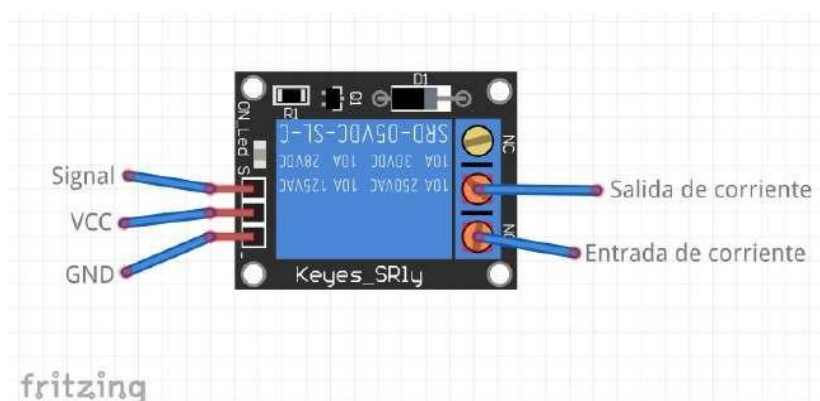
Figura 2. Conexiones del Arduino a relé, y de red pública a relé.
