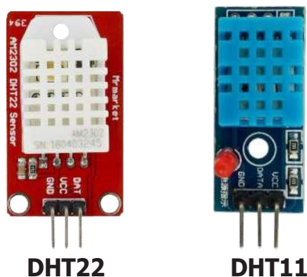
Figura 3.1. DHT22 y DHT11 indicando pines GND, 5V y Datos.
