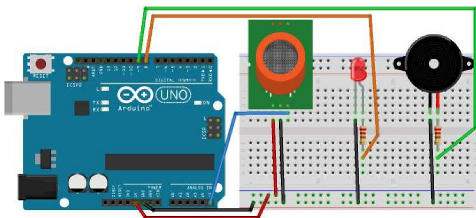
Figura 1. Circuito sensor de gas con alarma sonora.
