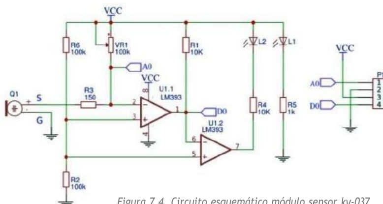
Figura 7.4. Circuito esquemático módulo sensor ky-037.
