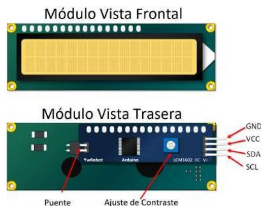
Figura 3. Componentes principales de display LCD con I2C.
