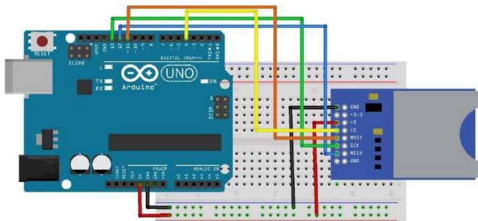
Figura 11.2. Esquema de conexión del Arduino a Breakout Board para tarjeta SD.
