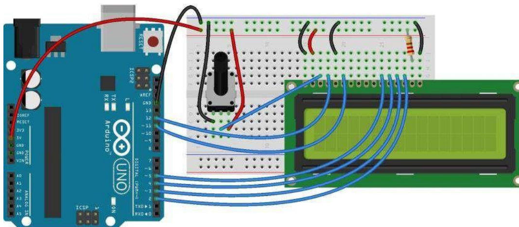
Figura 10.1. Esquema de circuito de display LCD conectado al Arduino UNO.
