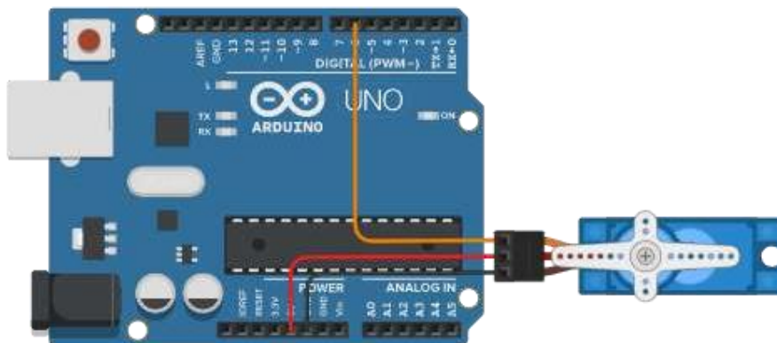
Figura 9.1. Modelo para el funcionamiento básico de un servomotor de giro restringido.
