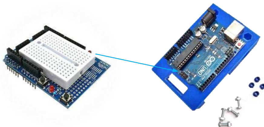
Figura 4. Paso 1: Montaje de placa Arduino UNO al cuerpo principal del chasis (vista superior), junto al Shield para prototipos.
