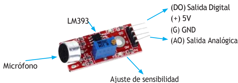
Figura 2. Componentes principales del módulo sensor ky-037.
