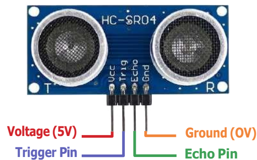
Figura 4. Componentes principales del módulo sensor ultrasónico HC-SR04.
