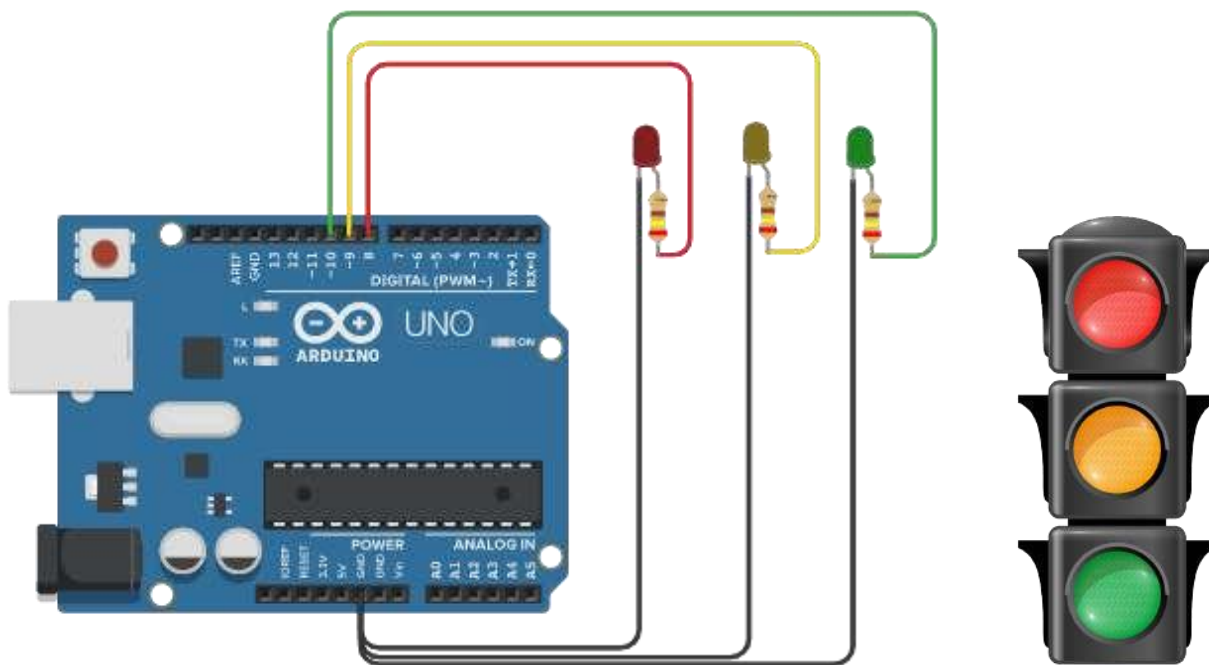
Figura 3.1. Circuito semáforo.
