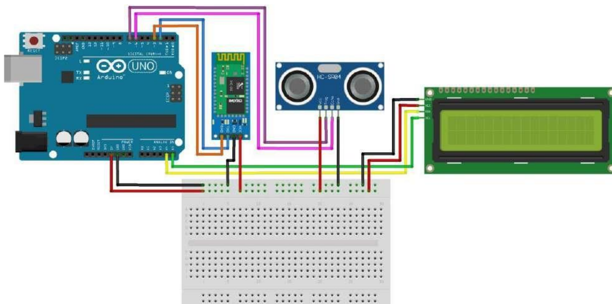
Figura 1. Esquema del circuito de regla digital.
