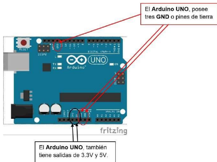
Figura 1.5: Tierras y salidas para alimentar led, sensores o pantalla LCD.
