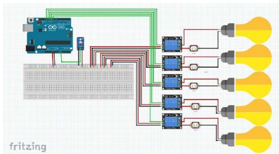
Figura 2. Esquema de circuito del solmáforo.
