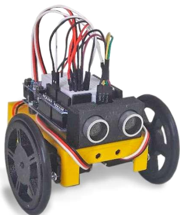
Figura 1. Robot LabTec armado completamente.
