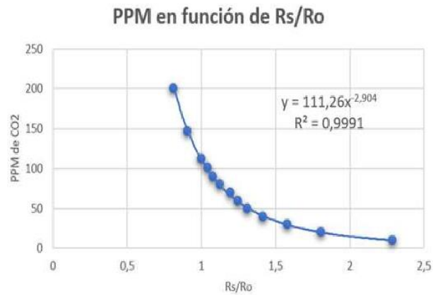
Figura 6. Curva característica del sensor MQ-135 y obtención de ecuación usando Excel.
