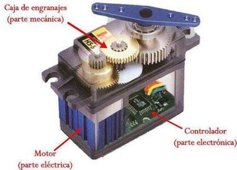
Figura 9.2. Componentes internas de un servomotor.
