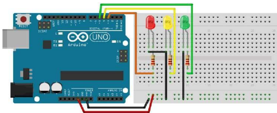
Figura 4. Circuito para el semáforo con LED.
