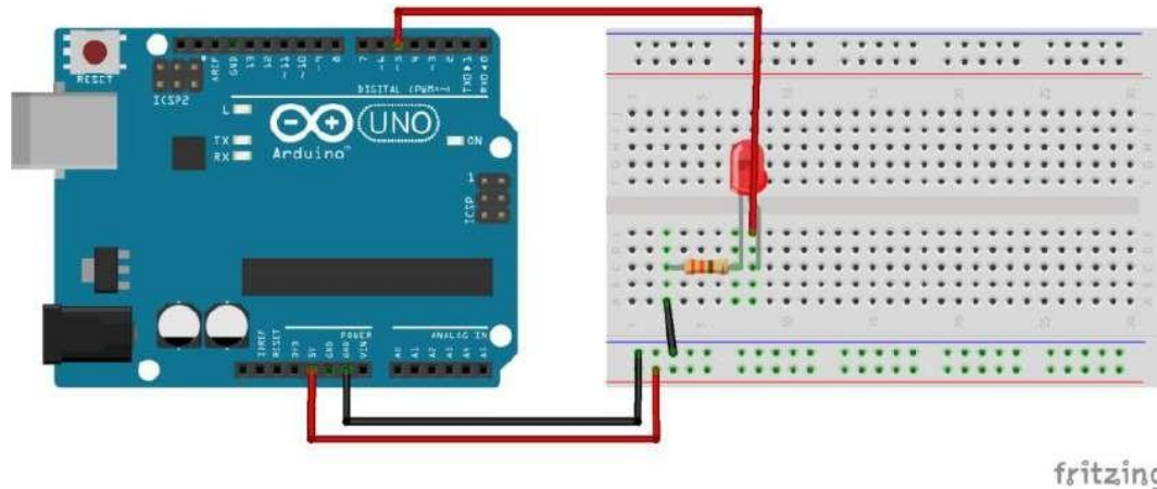
Figura 2.4. Conexión led-Arduino en pin digital 5.
