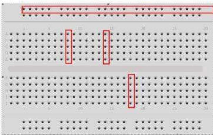
Figura 2.1. Protoboard indicando fila superior interconectada, y columnas también interconectadas según se indica en los rectángulos rojos.
