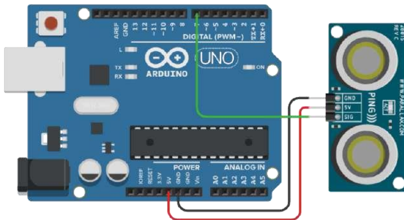
Figura 8.2. Montaje sensor ultrasónico PING))) desde Autodesk® Tinkercad®.
