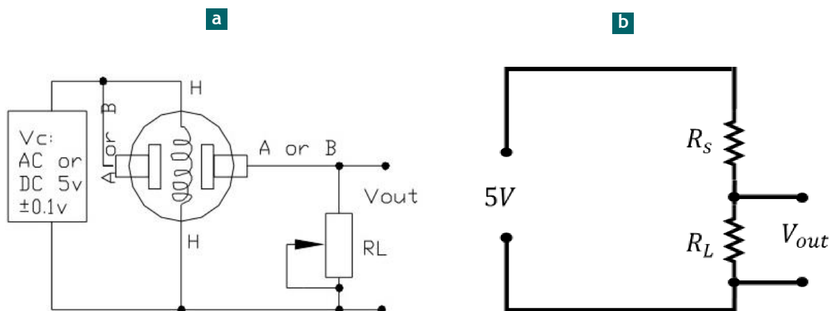
Figura 3. a) Circuito esquemático del sensor MQ-135. b) Esquema circuito equivalente.
