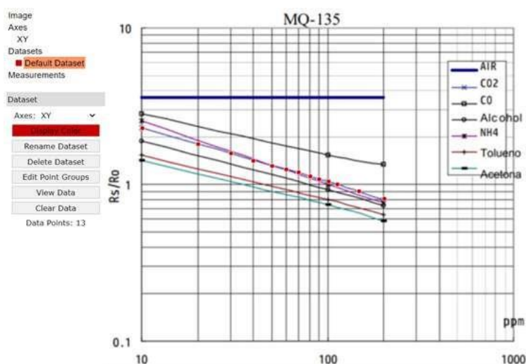
Figura 5. Curva característica del sensor MQ-135 y definición de puntos intermedios usando WebPlotDigitizer.
