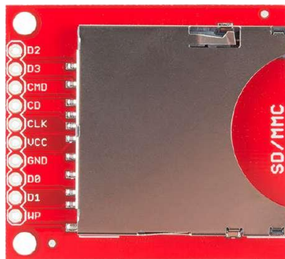
Figura 11.1. Breakout Board para tarjeta SD de Sparkfun.
