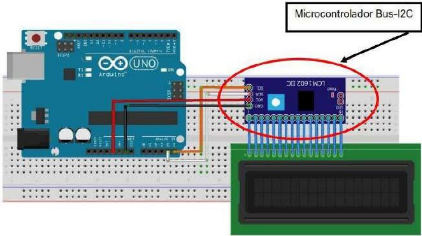
Figura 10.2. Esquema de circuito de display LCD de 16x2 con I2C, conectado al Arduino UNO.
