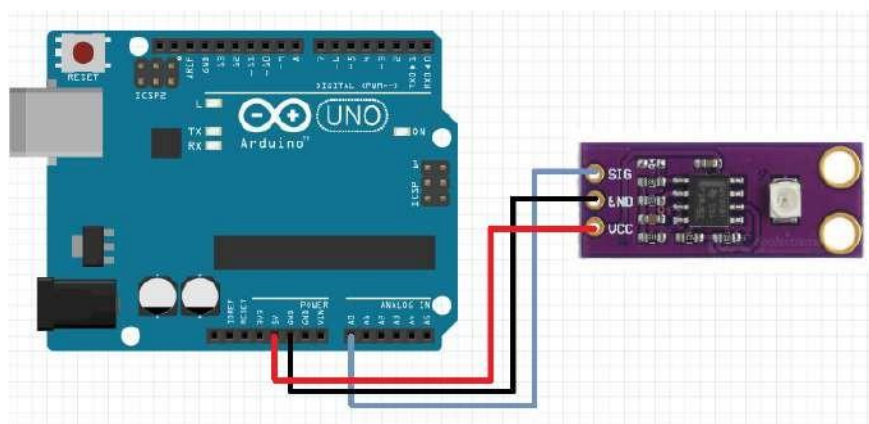
Figura 6.4: Conexión sensor UV GUA-S12SD con placa Arduino UNO.
