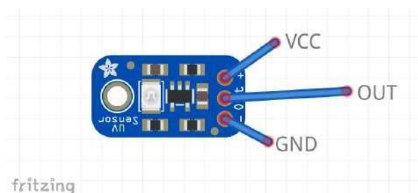
Figura 3. Componentes principales del sensor GUV S12SD.
