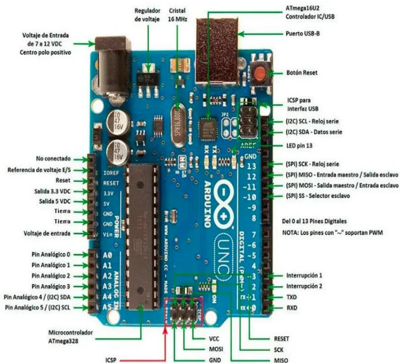
Figura 1.1: Arduino UNO esquematizado y partes importantes.
