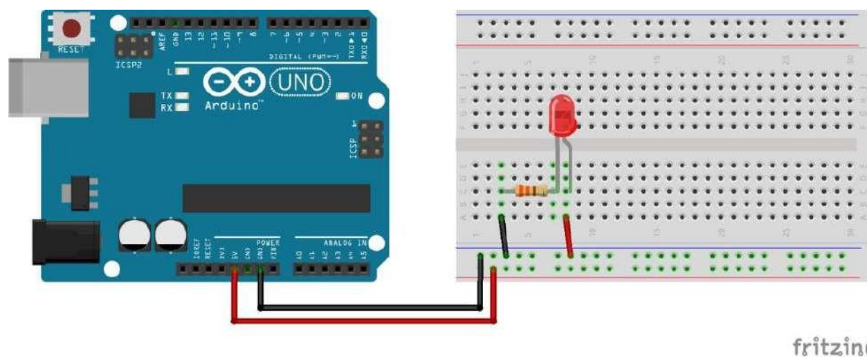
Figura 2.3. Conexión básica Arduino luz led.
