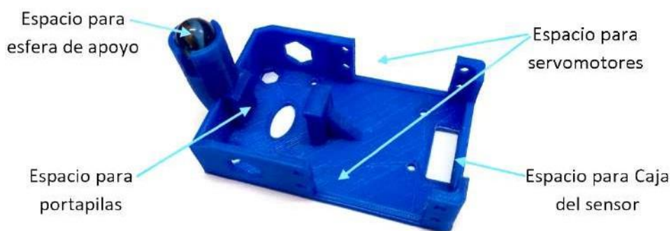
Figura 3. Cuerpo principal del chasis con detalle de sus partes (vista inferior).
