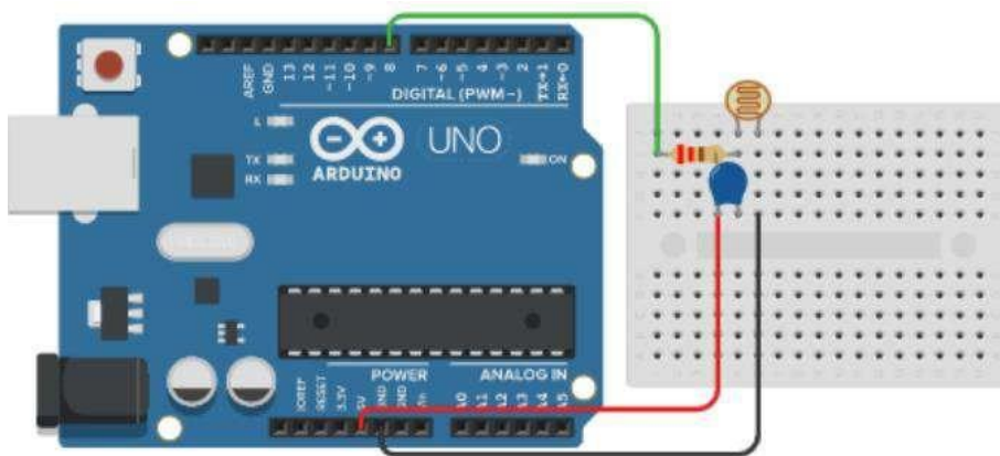
Figura 14.1. Circuito sensor PIR para activar un led.
