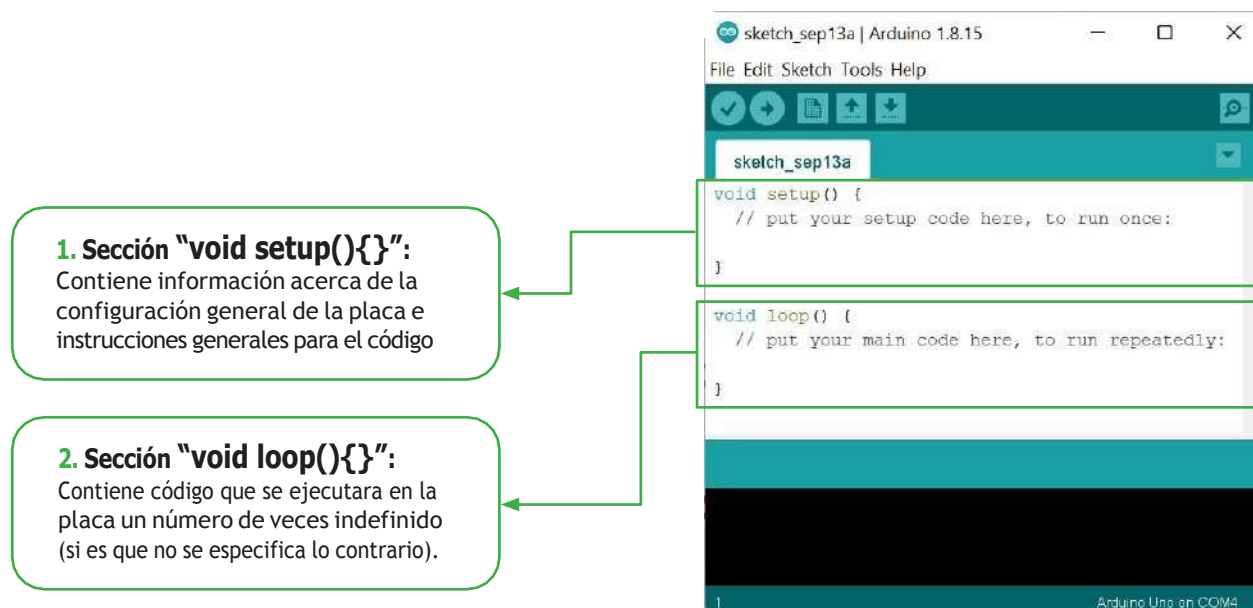
Figura 1.6: Entorno de programación IDE de Arduino.
